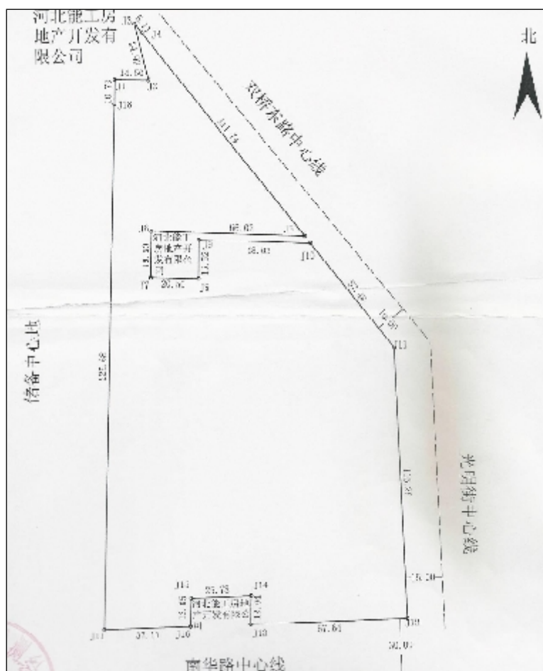
图 1-1 项目平面图
