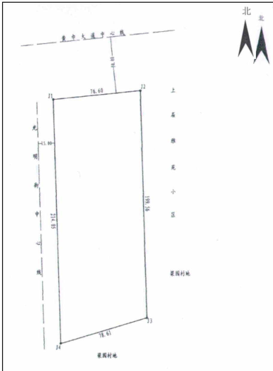
图 1-1 项目平面图
